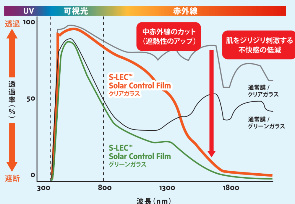
合わせガラスの光線透過率スペクトル比較 Comparison of light transmittance
