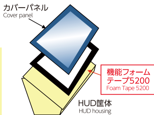
HUDカバーパネルの固定 Fixation of HUD Cover Panel
